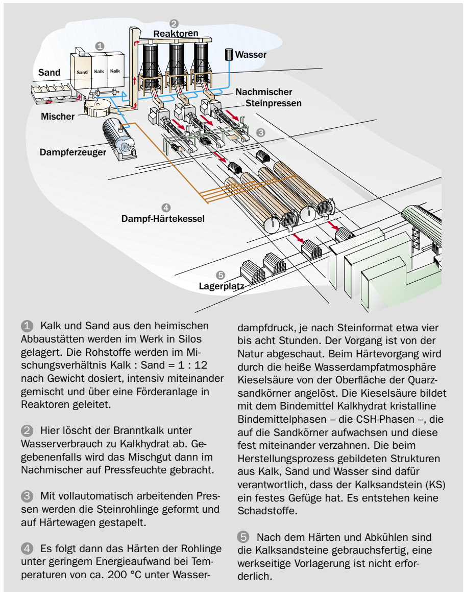
Bild 2/2: Die Herstellung von Kalksandstein [4].
