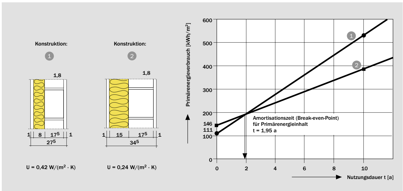
Bild 3/2: Amortisationszeit für Primärenergieverbrauch
