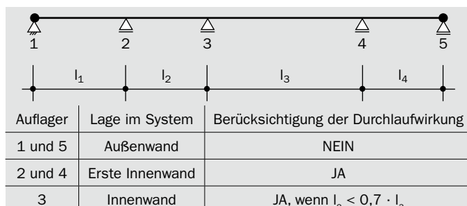
Bild 2/1: Ermittlung der Deckenaflagerkräfte bei einachsig gespannten Decken
